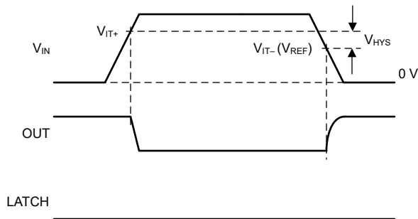
図 6-1. スwitchング スレッショルドとヒステリシス
