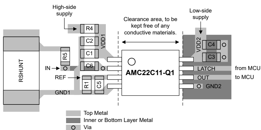
図 7-5. AMC22C11-Q1 の推奨レイアウト
