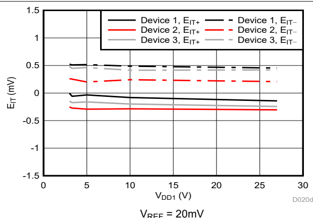
図 5-5. Cmp0 のトリップ・スレッシュホールド誤差と電源電圧との関係
