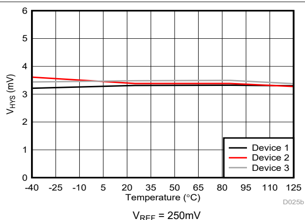
図 5-14. Cmp0 のトリップ・スレッシュホールドのヒステリシスと温度との関係
