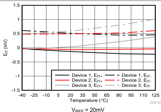
図 5-6. Cmp0 のトリップ・スレッシュホールド誤差と温度との関係
