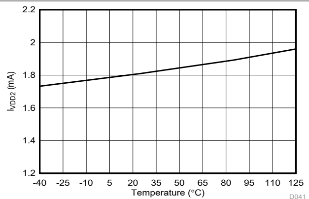
図 5-42. ハイサイド電源電流と温度との関係
