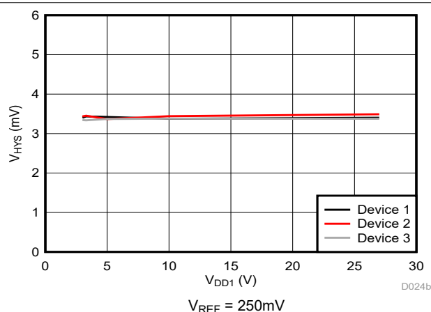
図 5-13. Cmp0 のトリップ・スレッシュホールドのヒステリシスと電源電圧との関係
