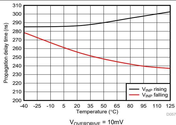
図 5-34. Cmp0 の伝搬遅延と温度との関係
