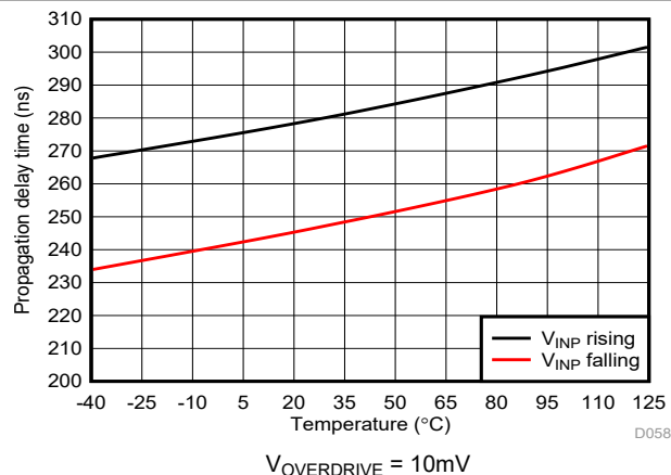
図 5-36. Cmp1 の伝搬遅延と温度との関係
