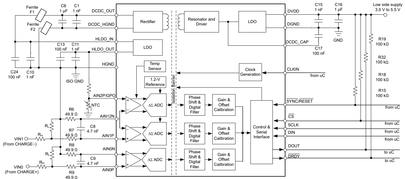
图 9-6. Power Supply Decoupling the AMC131M03-Q1
