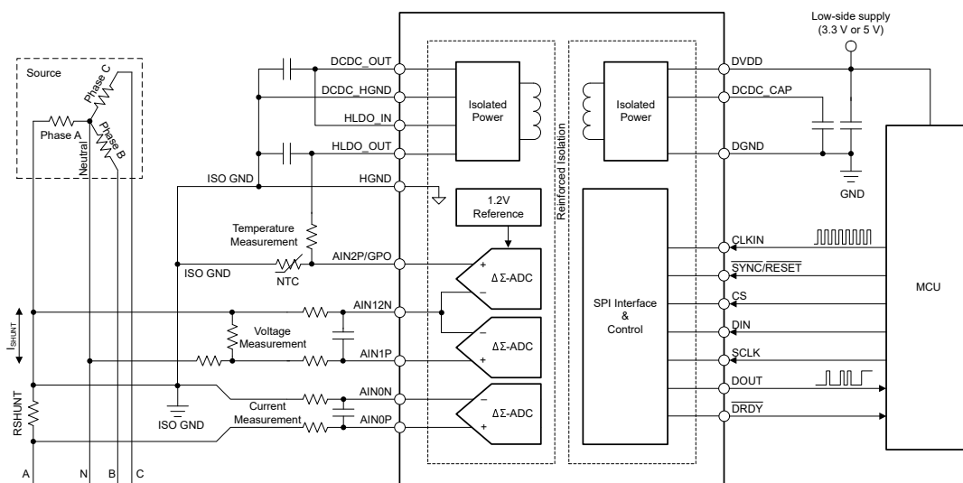
エネルギー・メーターにおける AMC131M03 の代表的なアプリケーション
