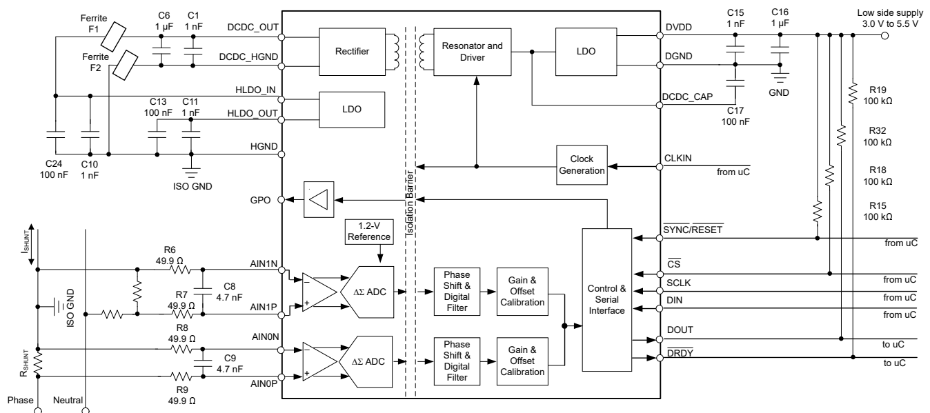
図 9-8. Power Supply Decoupling the AMC131M02
