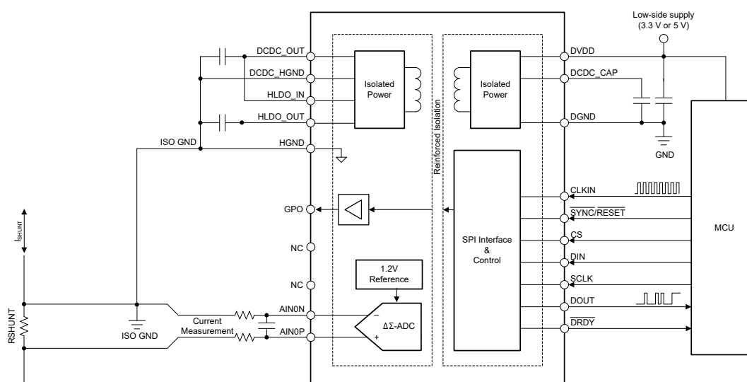
エネルギー・メーターにおける AMC131M01 の代表的なアプリケーション
