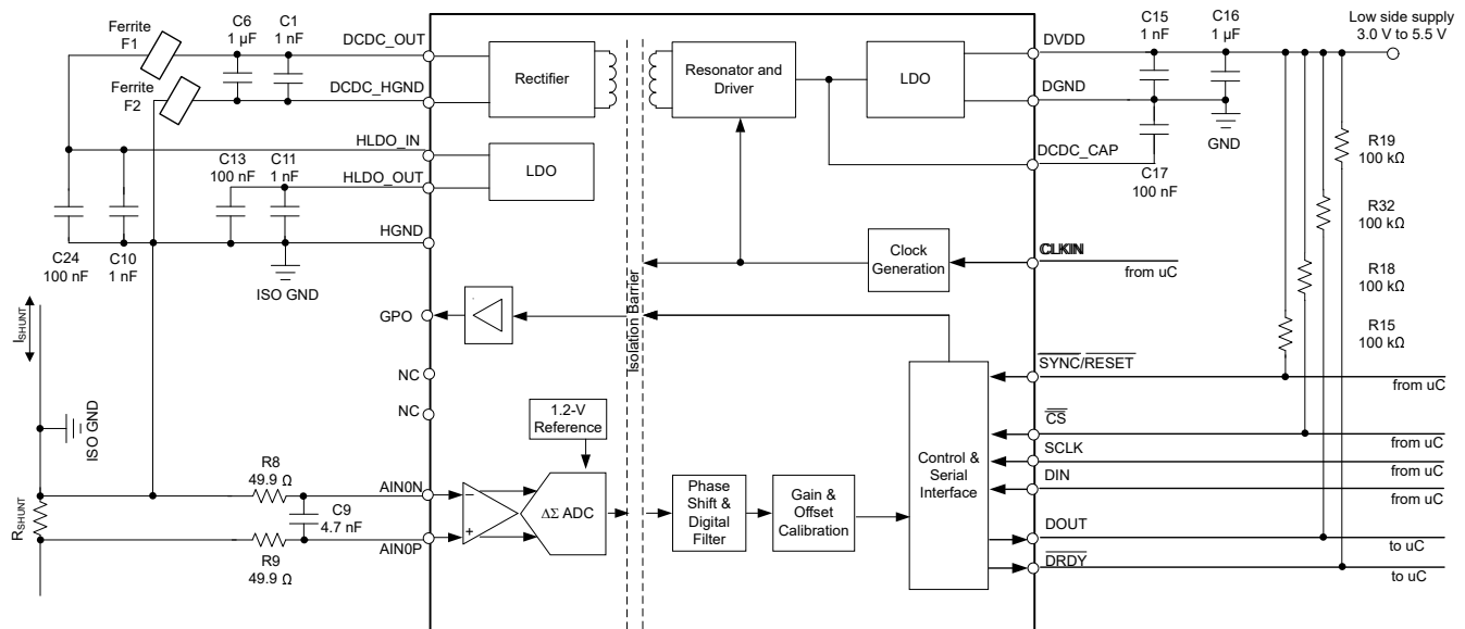
図 9-8. Power Supply Decoupling the AMC131M01
