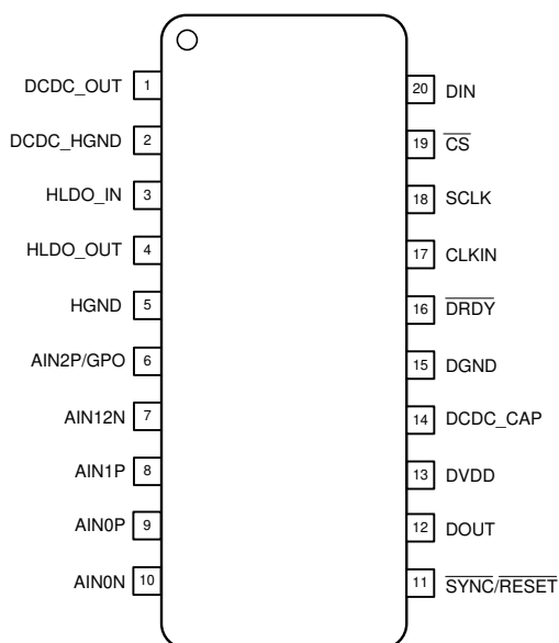
図 5-1. DFM Package, 20-Pin SOIC (Top View)
