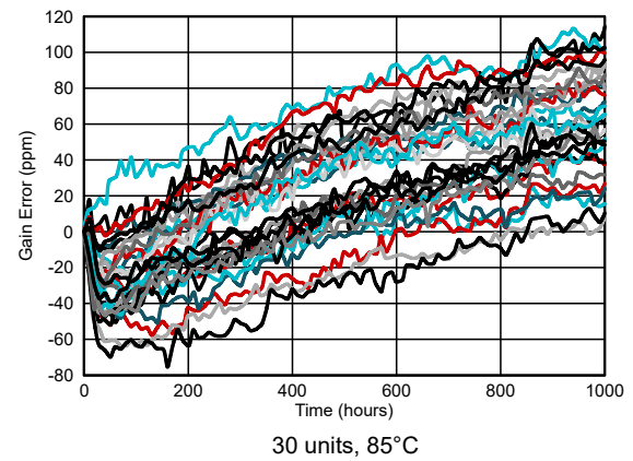
図 6-11. Gain Error vs Time
