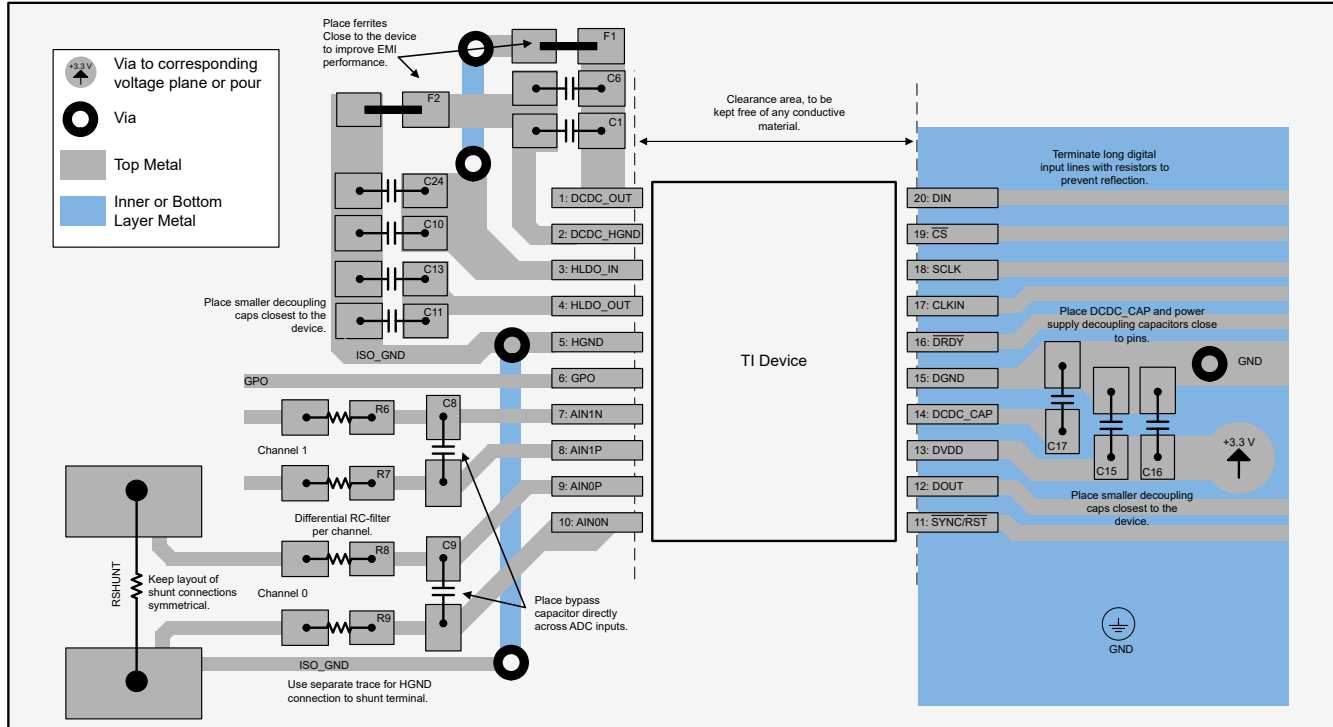
図 9-9. Layout Example
