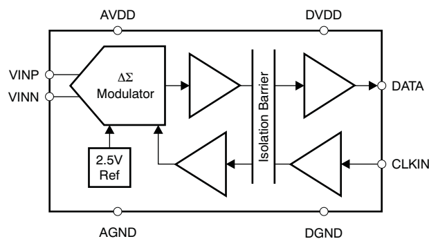
デバイスのブロック図
