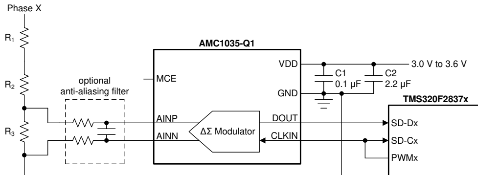
FIG 48. Decoupling the AMC1035-Q1
