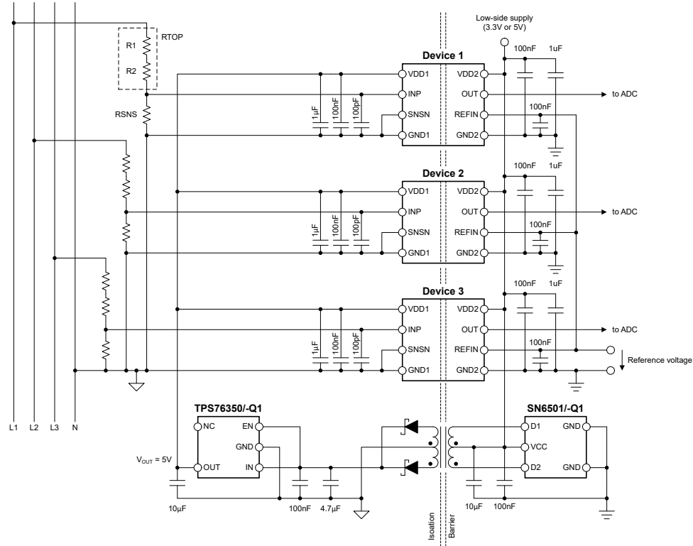
図 8-1. 代表的なアプリケーションで使用 AMC0x30S
