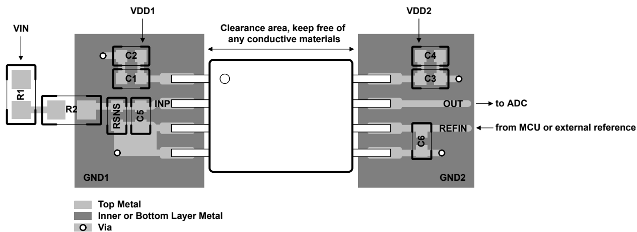
図 8-6. AMC0x11R
