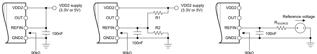
図 8-3. REFIN ピンに接続します
