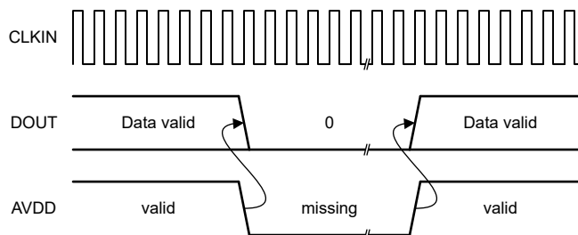
図 7-7. ハイサイド電源が消失した場合の AMC0x06M25 の出力
