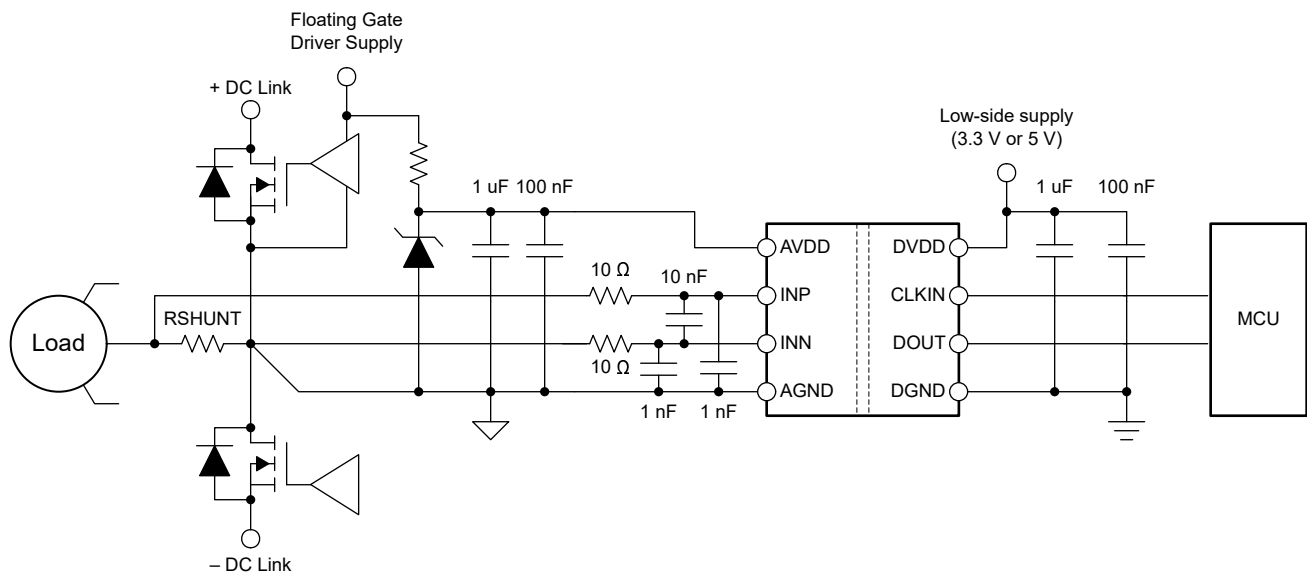
図 8-1. 代表的なアプリケーションでの電流検出に AMC0x06M25 を使用
