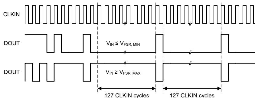
図 7-6. AMC0x06M25 のフルスケール出力
