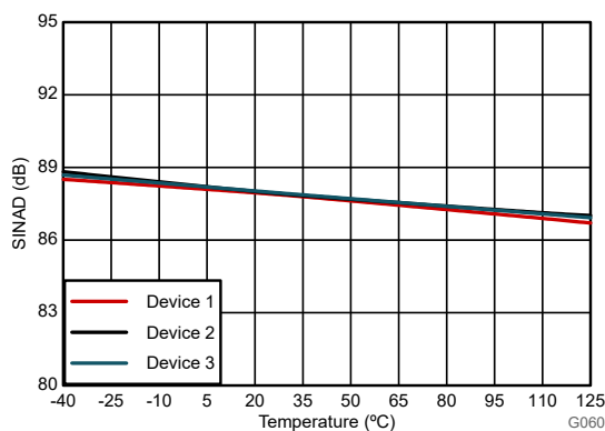
図 6-31. 信号対雑音比+歪みと温度との関係
