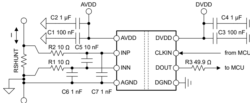
図 8-4. AMC0x06M25 のデカップリング
