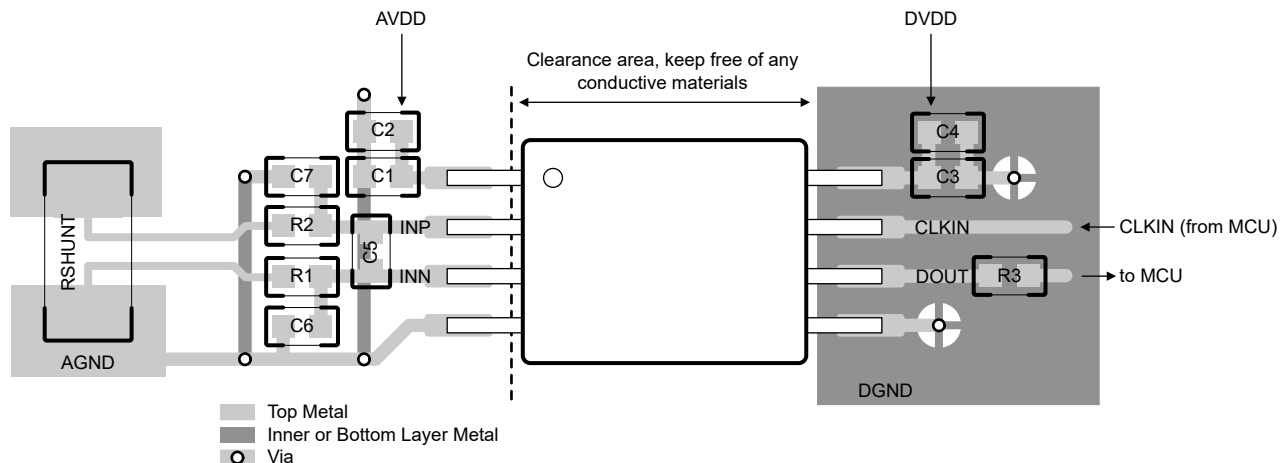
図 8-5. AMC0x06M05-Q1 の推奨レイアウト
