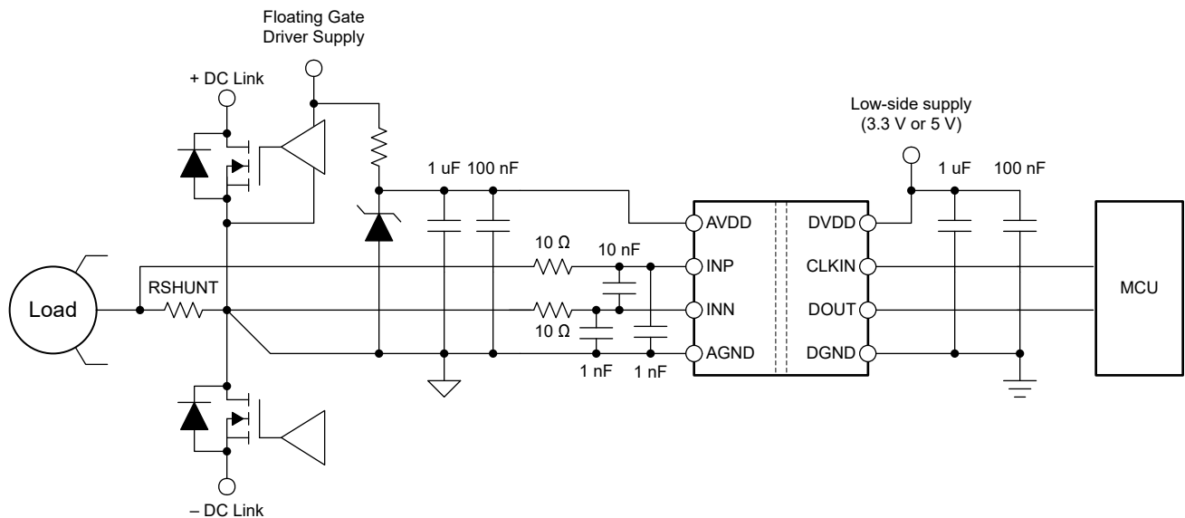
図 8-1. 代表的なアプリケーションでの電流検出に AMC0x06M05-Q1 を使用
