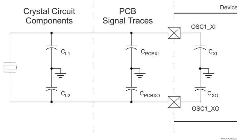
図 6-30. 負荷容量
