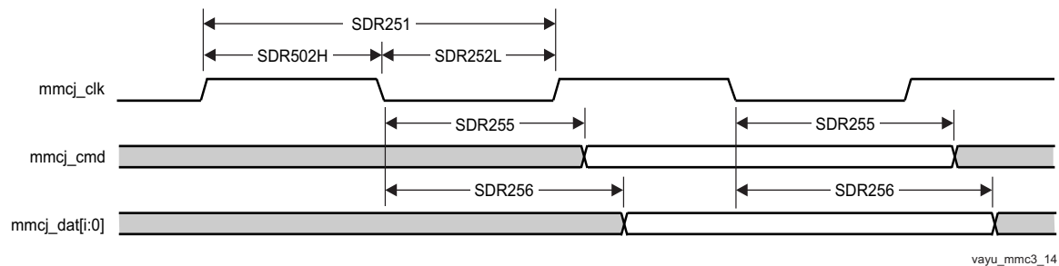
図 7-88. MMC/SD/SDIOj in - SDR25 - Transmitter Mode
