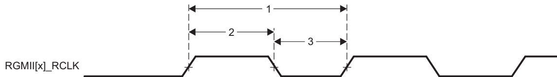
図 5-29. RGMII[x]_RCLK Timing - RGMII Mode
