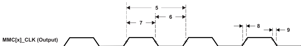
图 5-141. MMC[x]_CLK Timing
