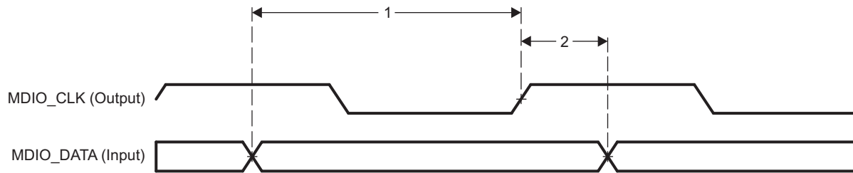
図 7-102. PRU-ICSS MDIO_DATA Timing - Input Mode
