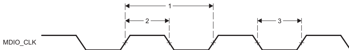
図 7-103. PRU-ICSS MDIO_CLK Timing
