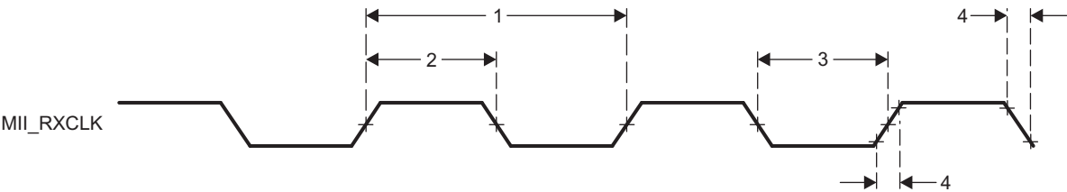
图 7-105. PRU-ICSS MII_RXCLK Timing
