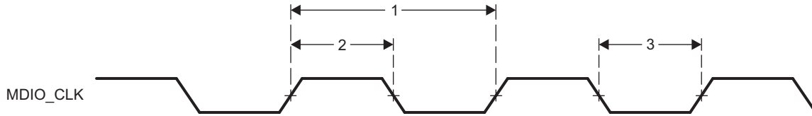
图 7-4. MDIO_CLK Timing
