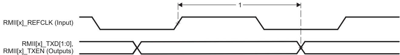
図 7-12. RMII[x]_TXD[1:0], RMII[x]_TXEN Timing - RMII Mode
