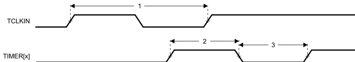
図 7-2. Timer Timing
