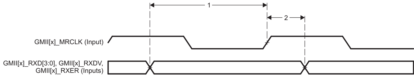
図 7-8. GMII[x]_RXD[3:0], GMII[x]_RXDV, GMII[x]_RXER Timing - MII Mode
