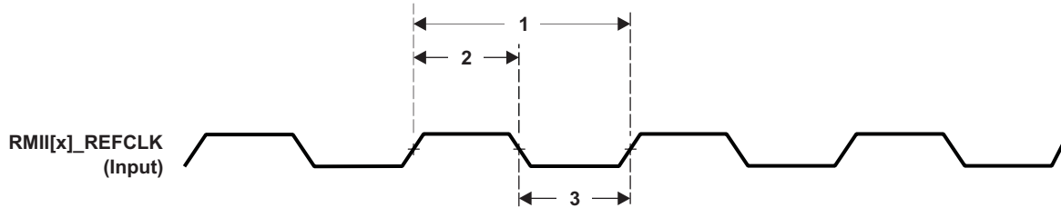
図 7-10. RMII[x]_REFCLK Timing - RMII Mode
