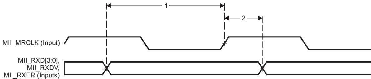
图 7-111. PRU-ICSS MII_RXD[3:0], MII_RXDV, and MII_RXER Timing
