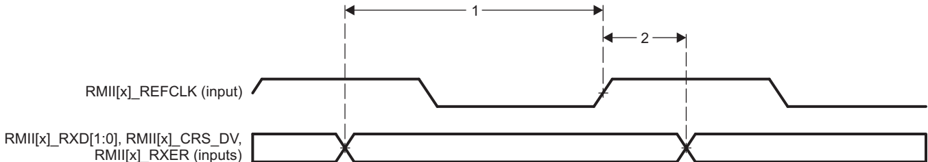
図 7-11. RMII[x]_RXD[1:0], RMII[x]_CRS_DV, RMII[x]_RXER Timing - RMII Mode
