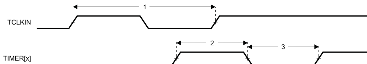
图 7-2. Timer Timing
