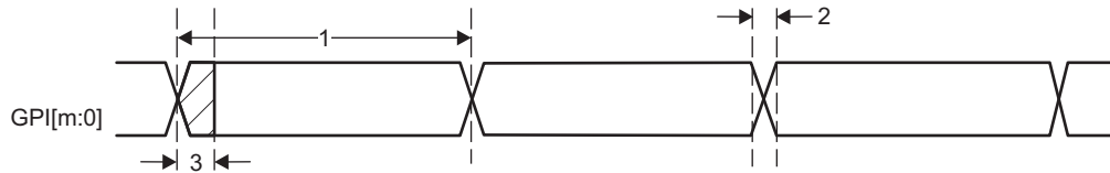
図 7-96. PRU-ICSS PRU Direct Input Timing
