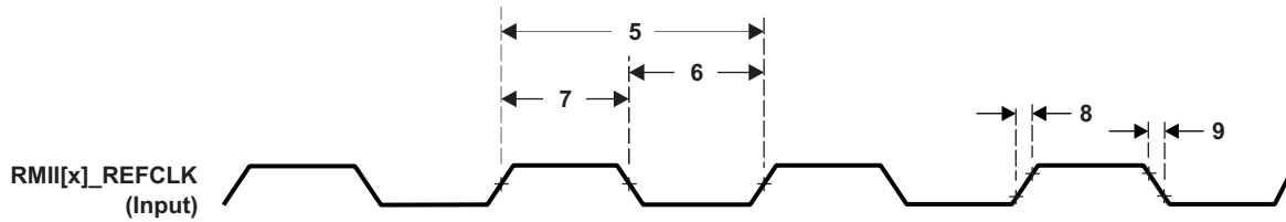
図 7-93. MMC[x]_CLK Timing
