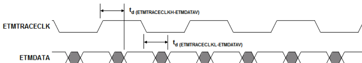
図 6-25. ETMDATA Timing
