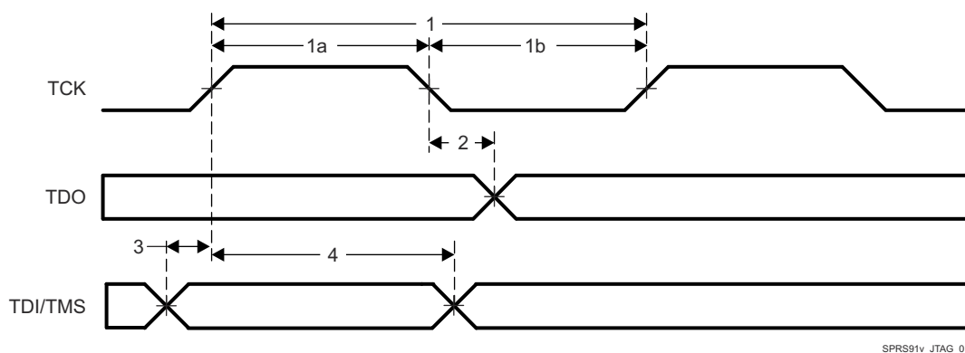
図 6-23. JTAG Timing
