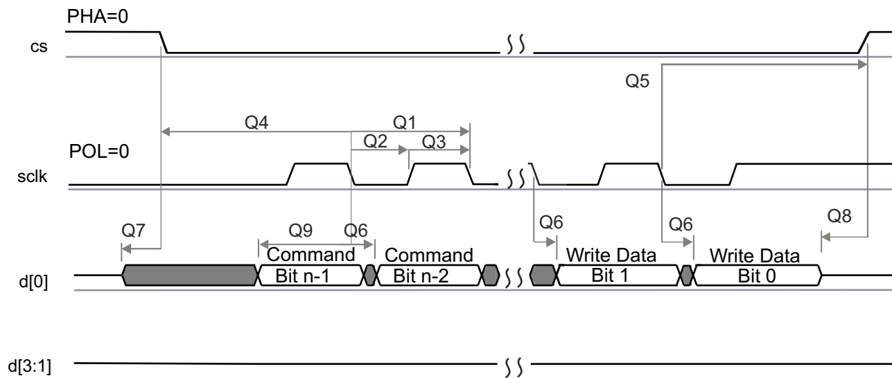
図 6-4. QSPI Write (Clock Mode 0)
