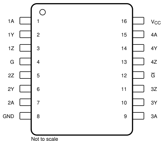
図 4-1. D or NS Package, SOIC 16 Pins (Top View)
