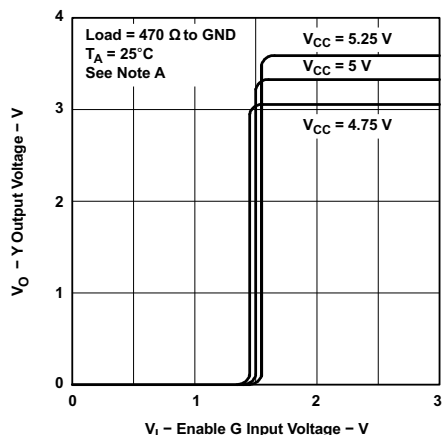
図 5-1. Output Voltage vs Enable G Input Voltage
