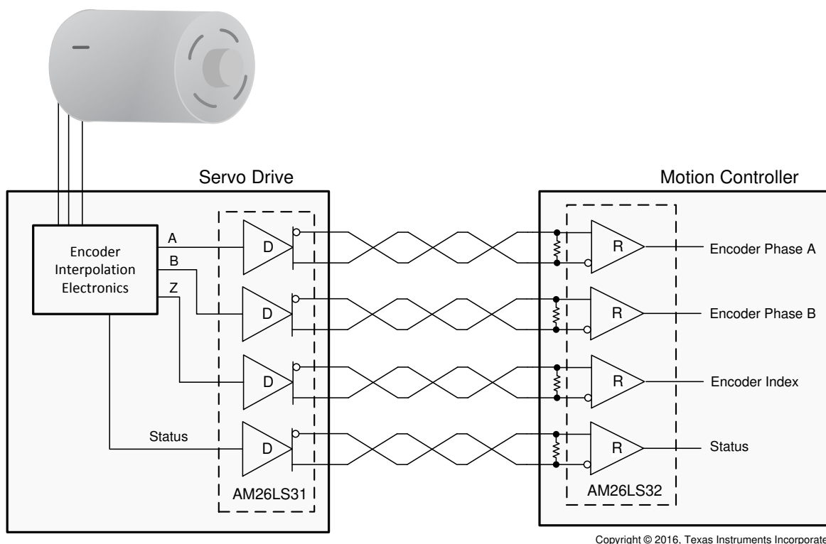
図 8-1. Encoder Application
