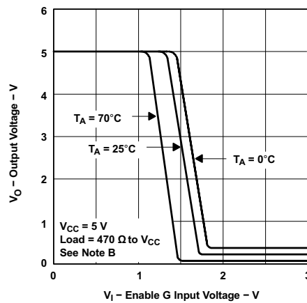
図 5-2. Output Voltage vs Enable G Input Voltage
