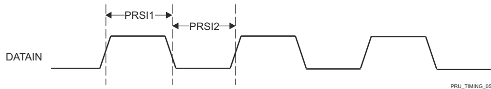
図 6-46. PRU-ICSS PRU Shift In Timing
