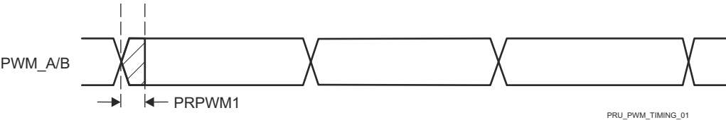
图 6-52. PRU-ICSS PWM Timing
