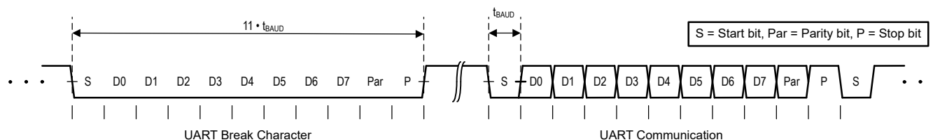
図 5-2. UBM Timing
