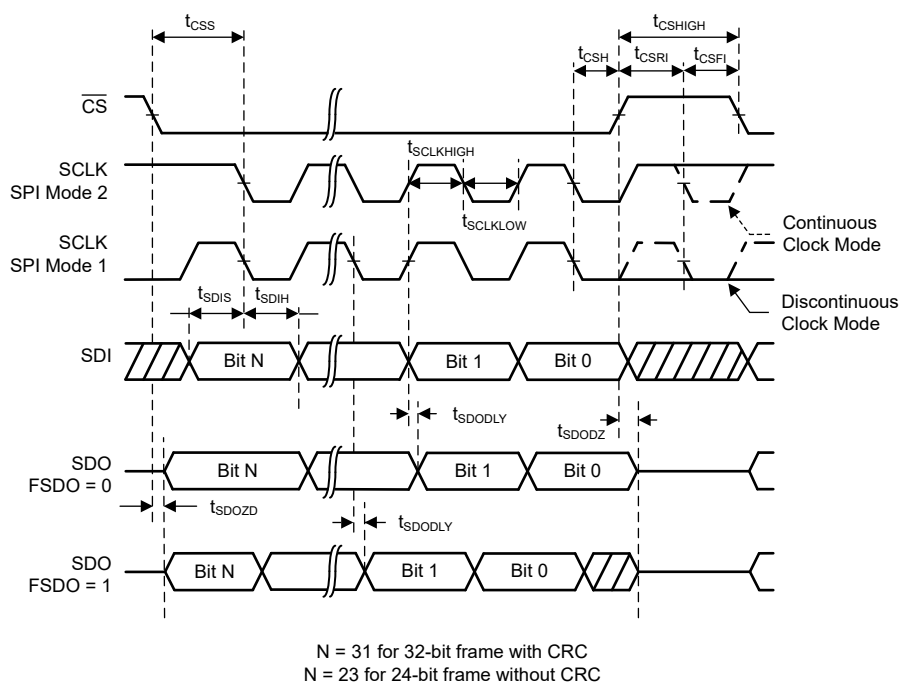
図 5-1. SPI Timing
