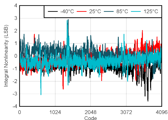
図 5-29. ADC INL vs Digital Input Code
