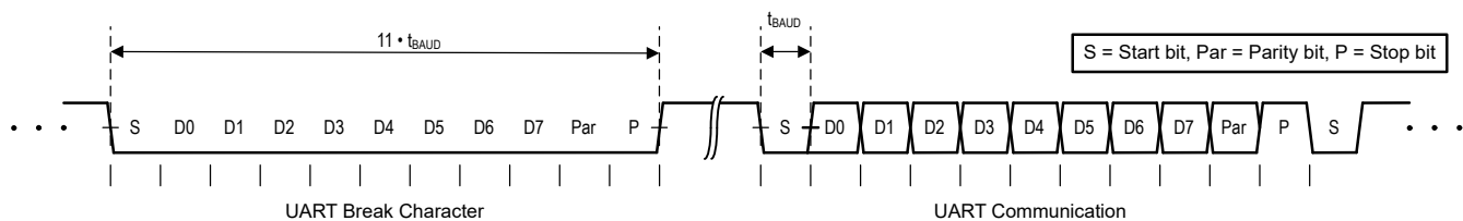
图 5-2. UBM Timing
