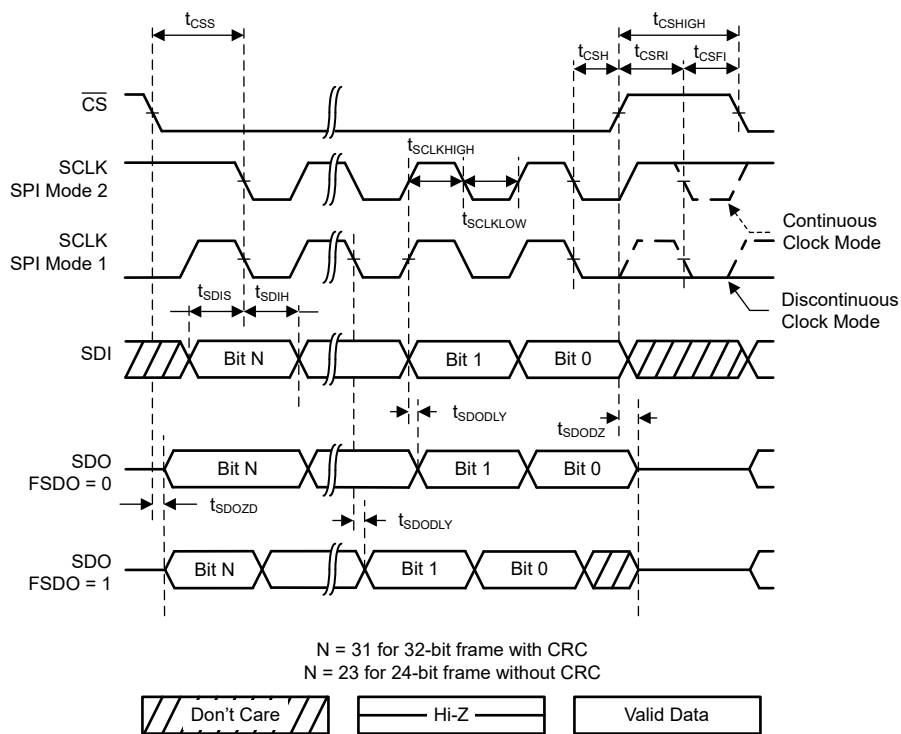
图 5-1. SPI Timing
