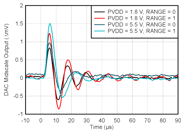
6-26. DAC Glitch Impulse Falling Edge
