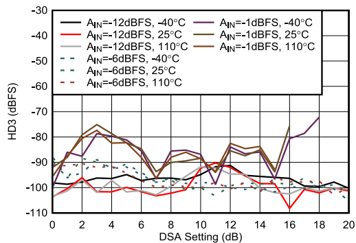
図 4-438. RX HD3 と DSA 設定との関係 (8.1GHz)
