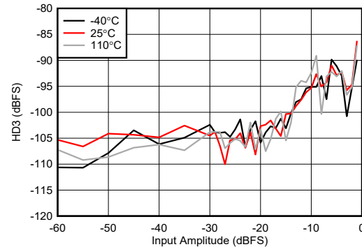
図 4-437. RX HD3 とデジタル振幅との関係 (8.1GHz)
