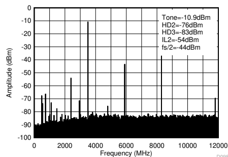
図 4-148. TX シングル トーン (-12dBFS) 出力スペクトル (0~ f_{\text{DAC}} 、3.5GHz)
