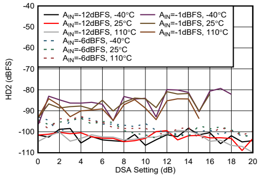
図 4-436. RX HD2 と DSA 設定との関係 (8.1GHz)
