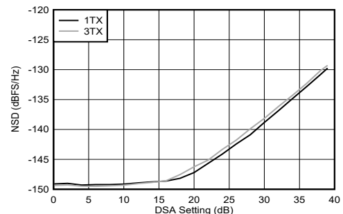
図 4-262. TX NSD と DSA 設定との関係 (9.61GHz)
