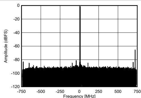
図 4-465. RX シングル トーン出力 FFT (9.61GHz)
