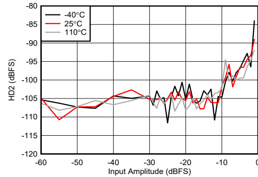
図 4-435. RX HD2 とデジタル振幅との関係 (8.1GHz)
