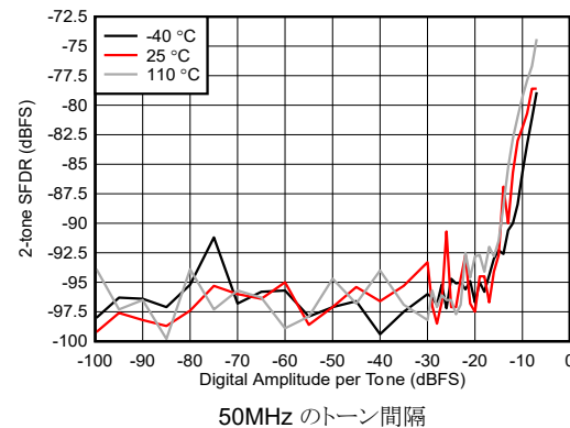
図 4-439. RX 2 トーン SFDR とデジタル振幅との関係 (8.1GHz)
