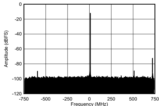
図 4-465. RX シングル トーン出力 FFT (9.61GHz)
