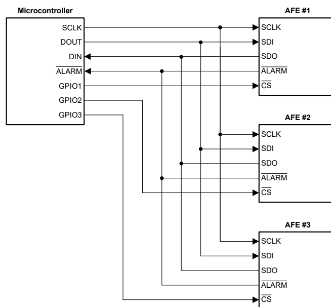
図 8-1. Multichannel Configuration
