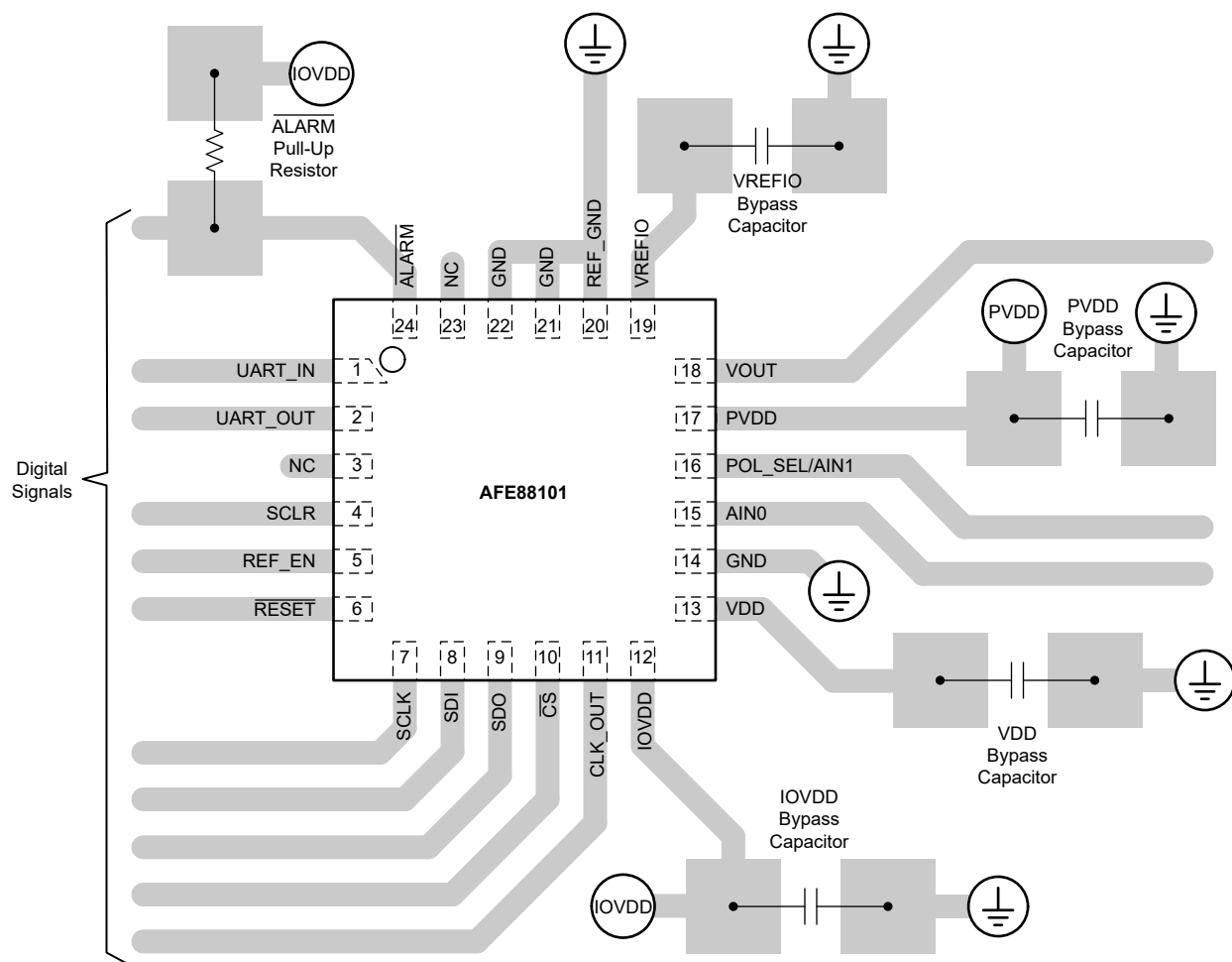
图 8-8. Layout Example
