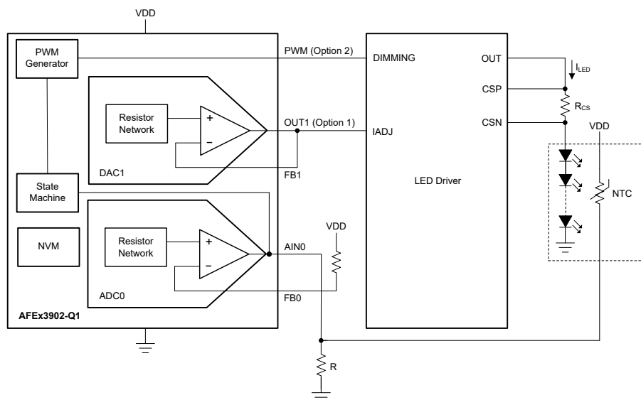
AFEx3902-Q1 を使用したマルチスロープ・サーマル・フォールドバック
