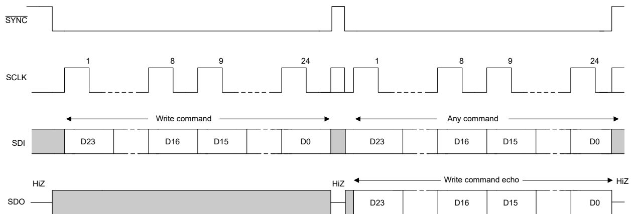
図 7-6. SPI Write Cycle
