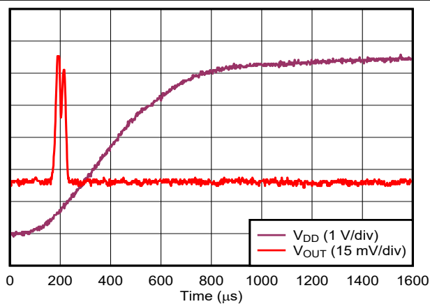
图 6-24. Voltage Output Power-On Glitch
