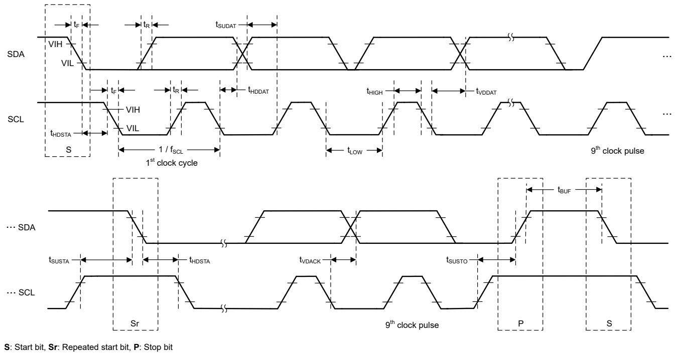
图 6-1. I²C Timing Diagram
