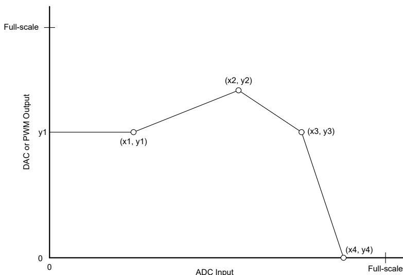
図 7-4. Multislope Transfer Function
