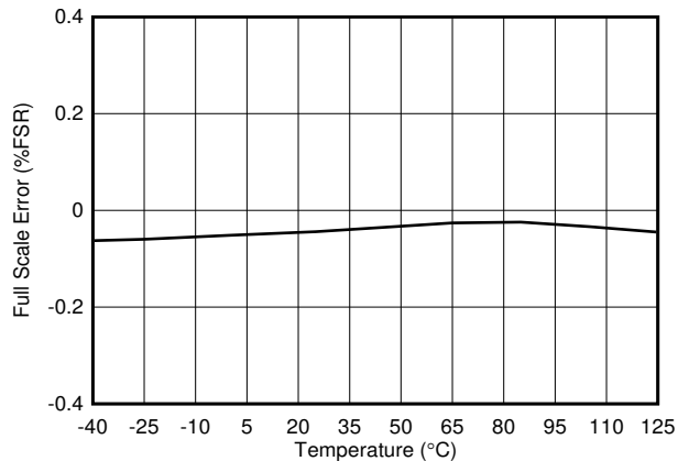
図 5-11. DAC ゲイン誤差と温度との関係
