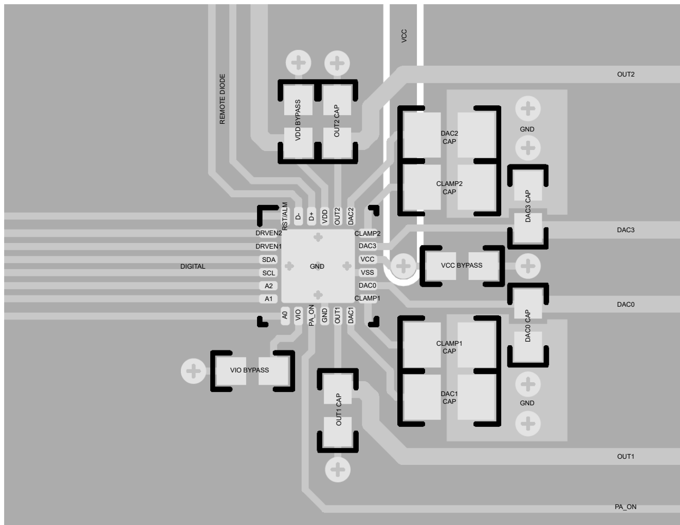
図 8-12. 正の出力のレイアウト例
