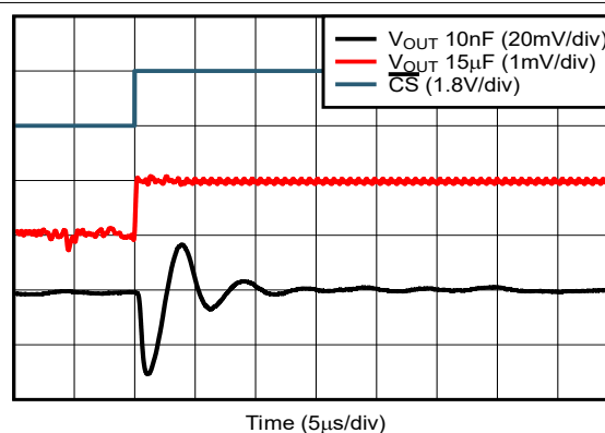
図 5-25. DAC グリッチ インパルス
