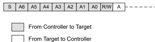
図 6-20. ターゲット アドレス アライメント
