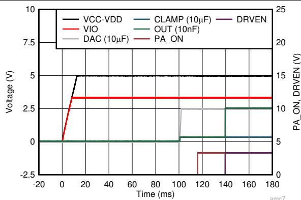
図 5-37. OUT ピン : CLAMP から DAC スwitchの応答
