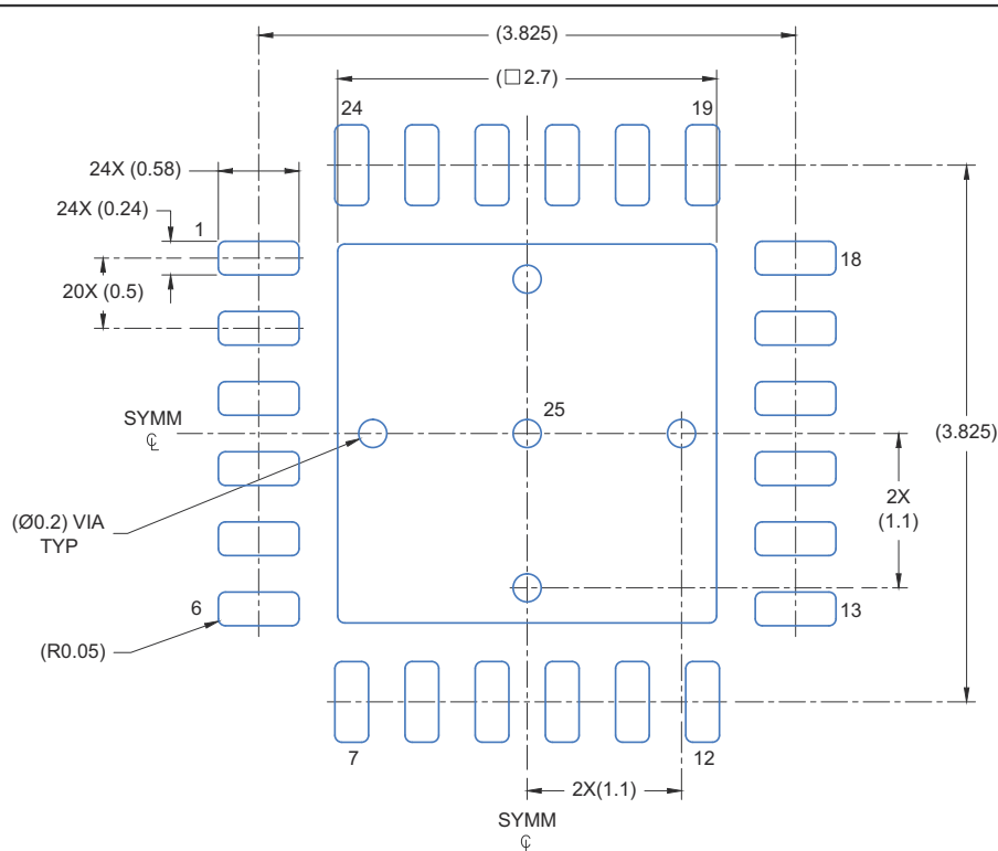
LAND PATTERN EXAMPLE SCALE: 20X
