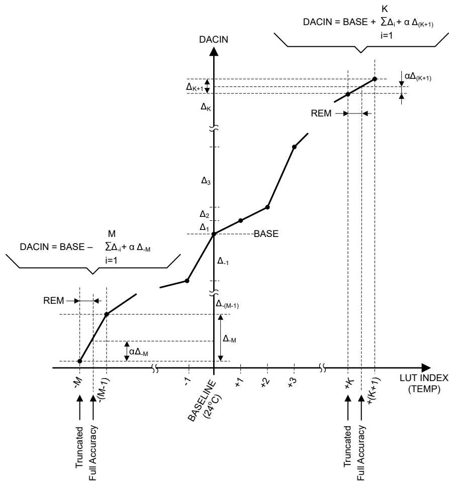
図 6-10. DACIN の計算
