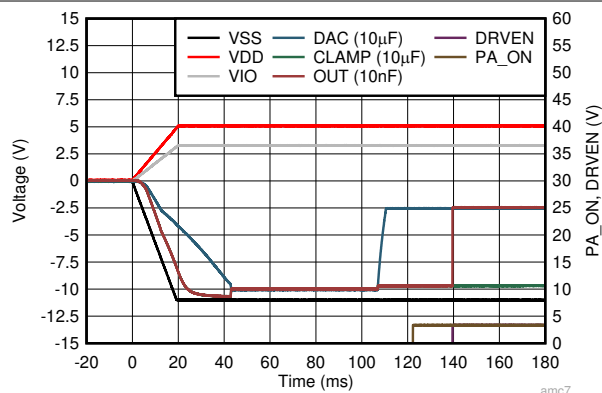
図 5-36. OUT ピン : CLAMP から DAC スwitchの応答
