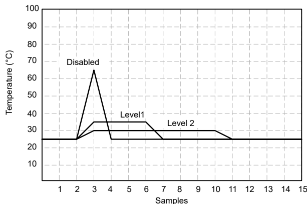
図 6-5. インパルス入力に対するフィルタ応答
