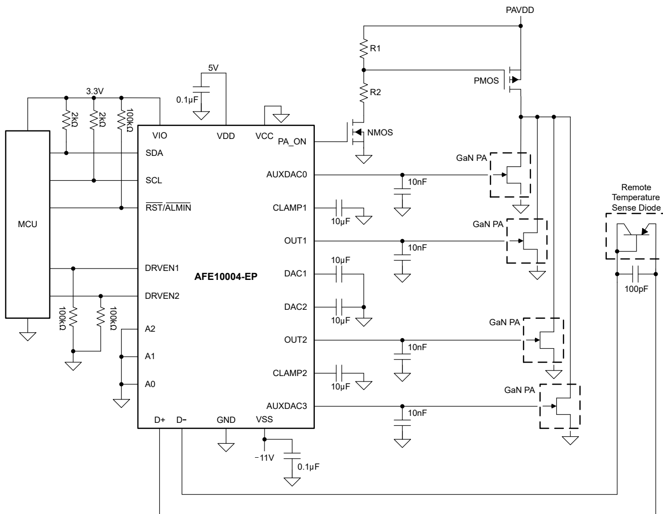
図 8-10. 代表的な GaN アプリケーション
