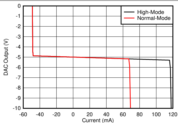
図 5-23. ソースおよびシンク電流能力
