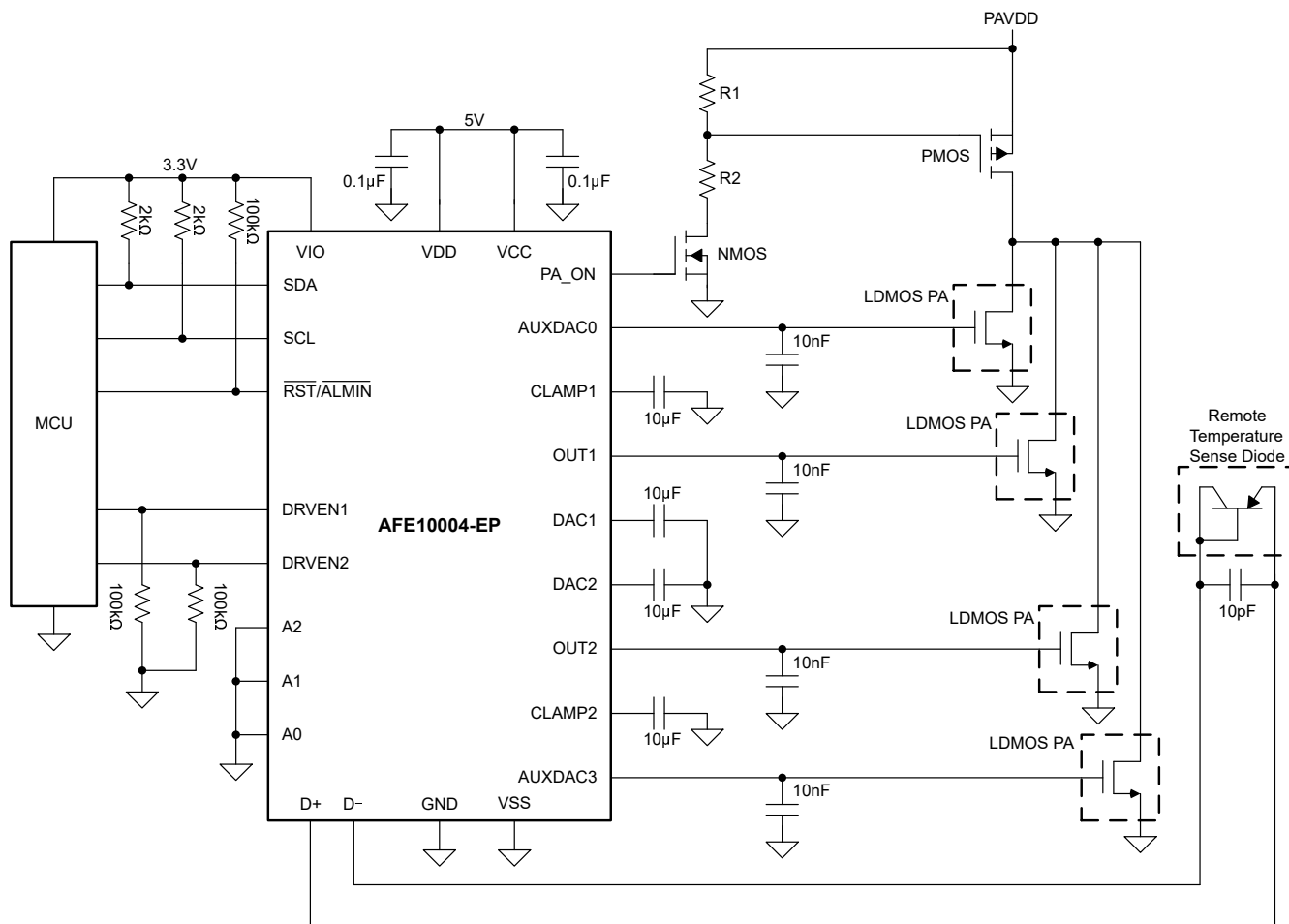
図 8-7. 代表的な LDMOS アプリケーション
