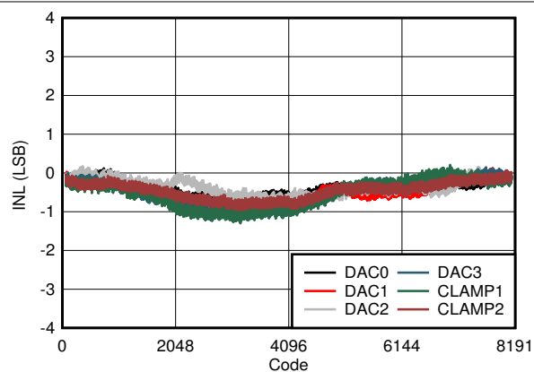
図 5-5. DAC INL とデジタル入力コードとの関係
