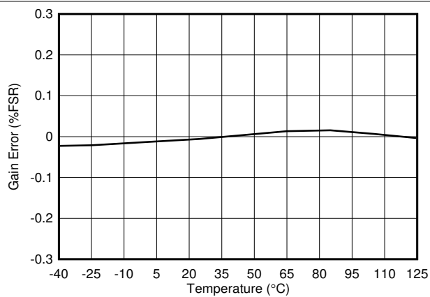
図 5-11. DAC ゲイン誤差と温度との関係
