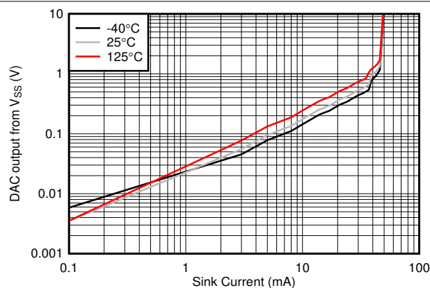
図 5-22. DAC[0:3] ヘッドルームと High モードシンキング電流の関係
