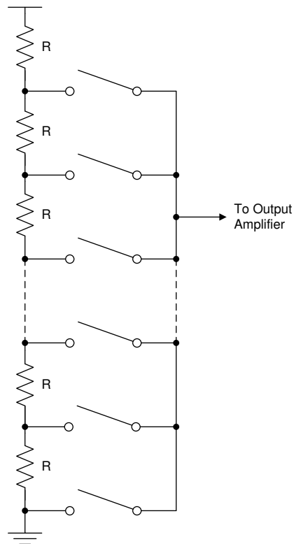
図 6-2. DAC 抵抗列
