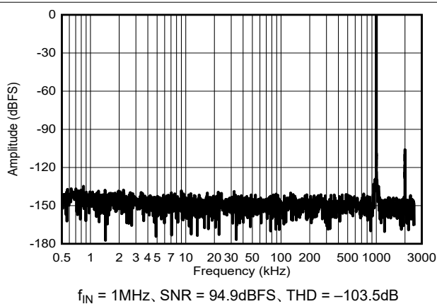
図 6-34. f_{IN} = 1\text{MHz} の標準 FFT
