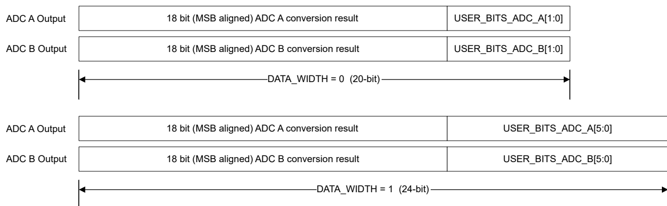
図 7-9. LSB XOR が有効な場合のデータ フレーム幅の構成
