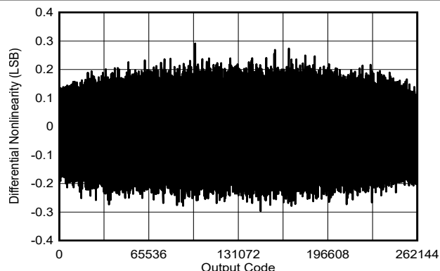
図 6-20. 標準 DNL
