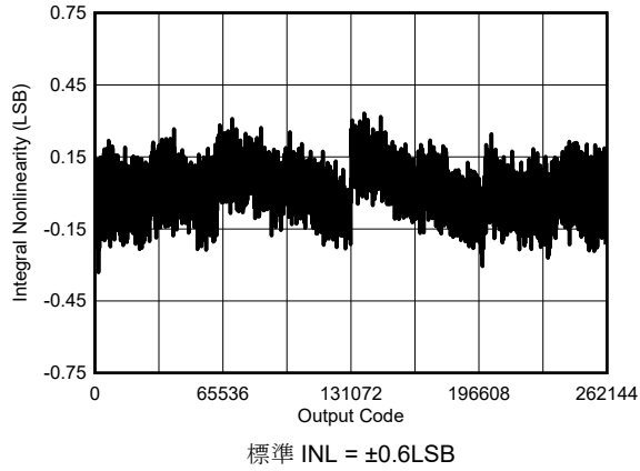
図 6-30. 標準 INL
