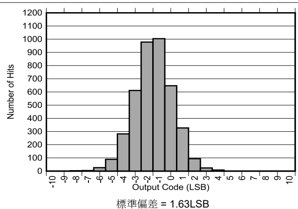
図 6-29. DC 入力ヒストグラム
