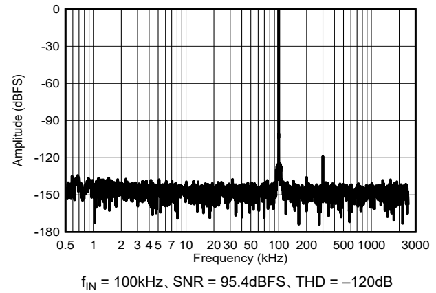
図 6-33. f_{IN} = 100\text{kHz} の標準 FFT
