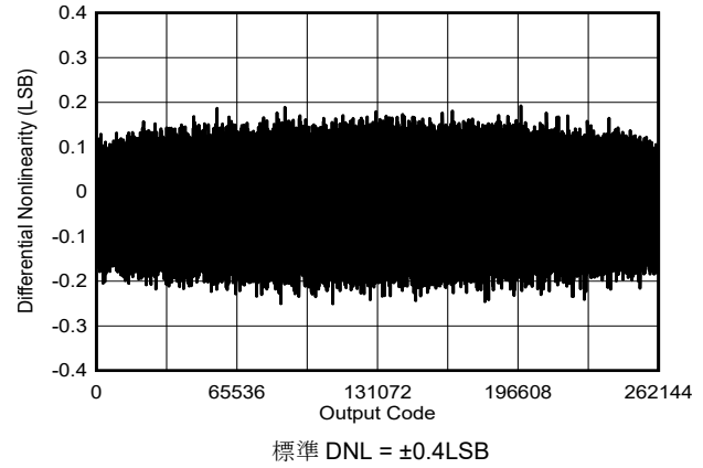
図 6-31. 標準 DNL
