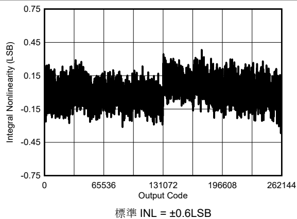
図 6-24. 標準 INL
