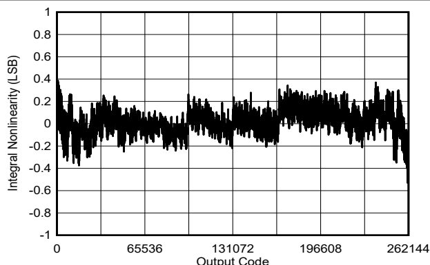
図 6-19. 標準 INL
