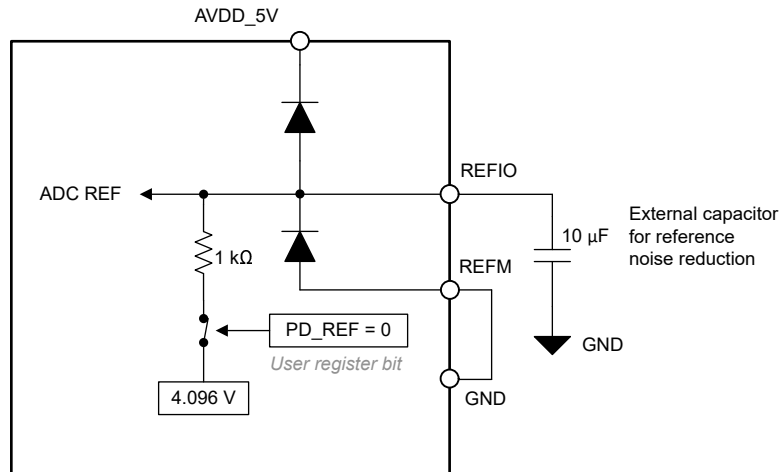
図 7-2. 内部リファレンス電圧
