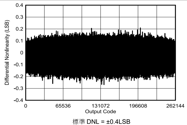
図 6-25. 標準 DNL
