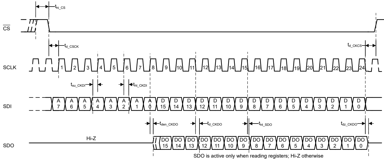
図 6-6. 構成 SPI
