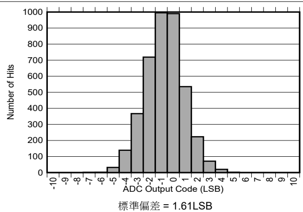
図 6-35. DC 入力ヒストグラム
