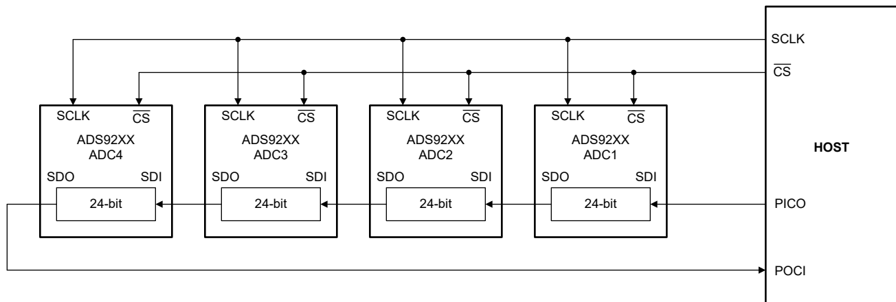
図 7-15. SPI 構成のデージーチェーン接続
