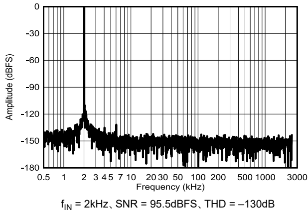
図 6-32. f_{IN} = 2\text{kHz} の標準 FFT
