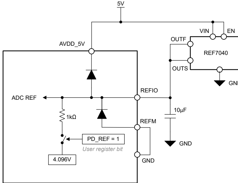
図 6-7. External Reference Voltage
