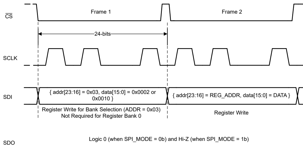
图 6-10. Register Write
