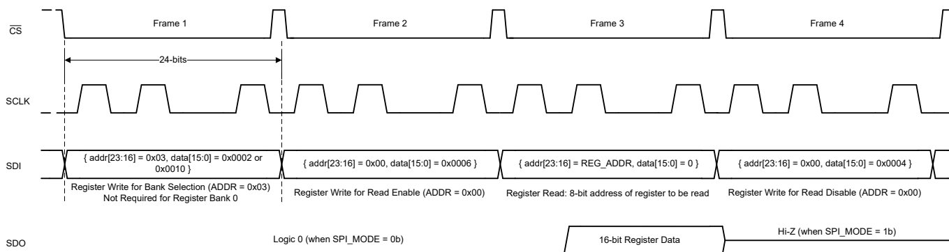
图 6-11. Register Read
