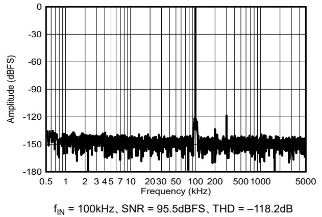
図 6-25. f_{IN} = 100\text{kHz} の標準 FFT
