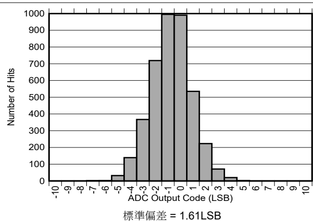
図 6-33. DC 入力ヒストグラム
