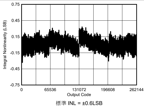
図 6-28. 標準 INL
