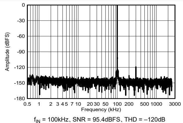
図 6-31. f_{IN} = 100\text{kHz} の標準 FFT
