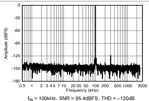
図 9-6. 5MSPS/チャンネルでの標準 FFT : ADS9117
