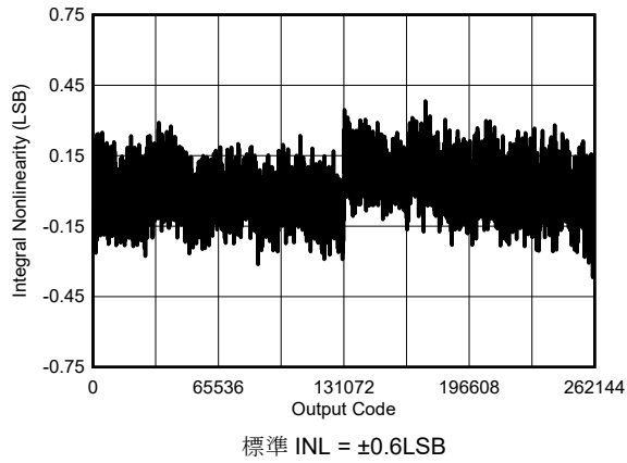
図 6-22. 標準 INL
