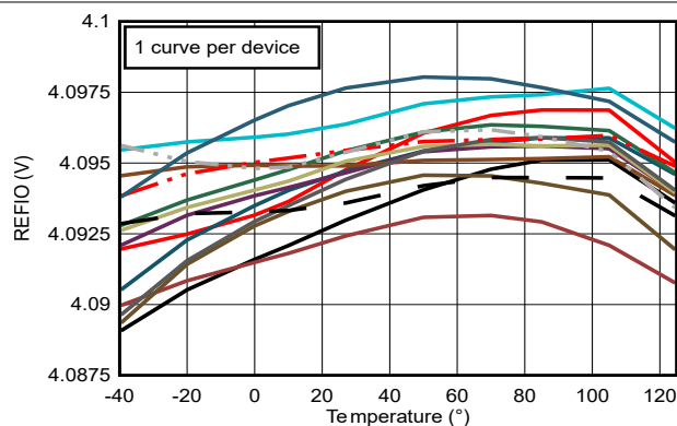
図 6-13. REFIO 電圧と温度との関係
