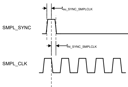
図 6-5. SMPL_SYNC タイミング
