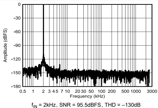
図 6-30. f_{IN} = 2\text{kHz} の標準 FFT
