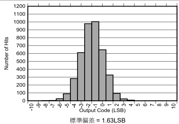
図 6-27. DC 入力ヒストグラム
