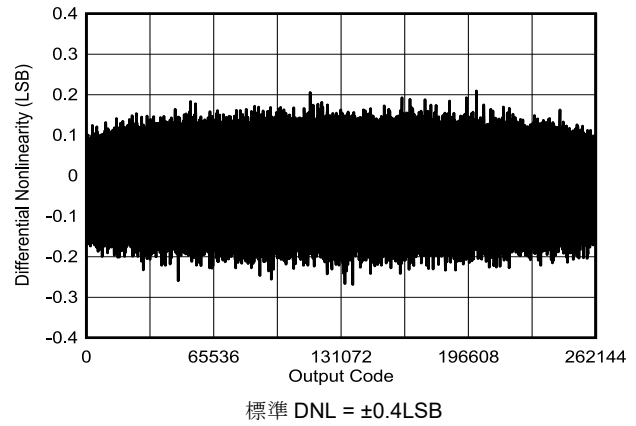
図 6-23. 標準 DNL
