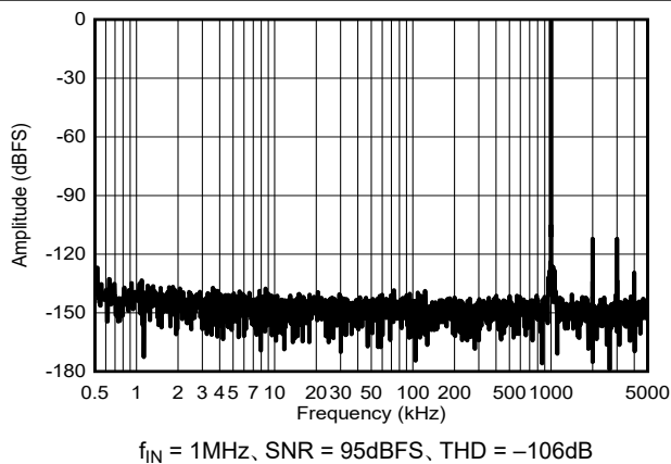
図 6-26. f_{IN} = 1\text{MHz} の標準 FFT
