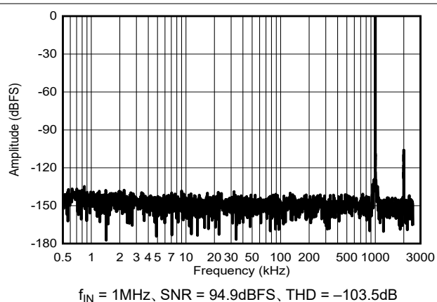
図 6-32. f_{IN} = 1\text{MHz} の標準 FFT
