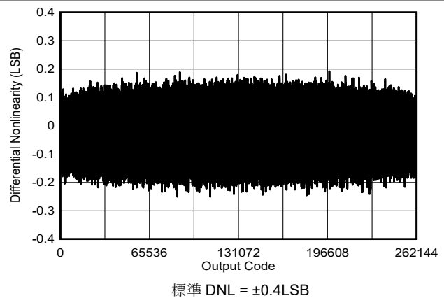
図 6-29. 標準 DNL
