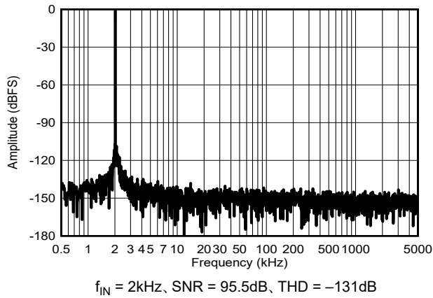
図 6-24. f_{IN} = 2\text{kHz} の標準 FFT
