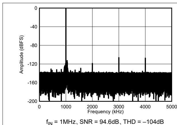
図 9-8. 10MSPS/チャンネルでの標準 FFT : ADS9118
