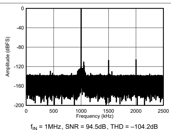
図 9-9. 5MSPS/チャンネルでの標準 FFT : ADS9117
