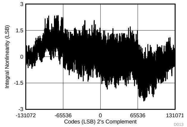
FIG 17. INL vs All Codes ( \pm 10\text{ V} )
