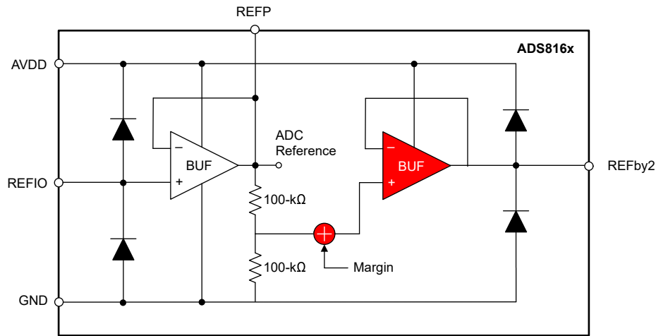
6-9. REFby2 Buffer Model
