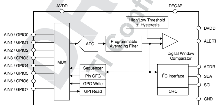
ADS7138-Q1 のブロック図とアプリケーション
