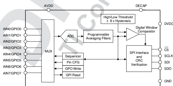
ADS7038-Q1 のブロック図とアプリケーション
