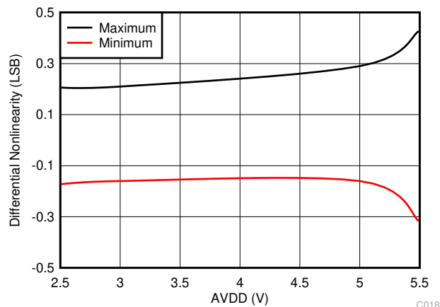
FIG 7-9. DNL vs AVDD
