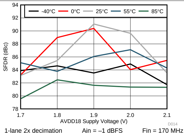
Figure 18. SFDR vs. AVDD18
