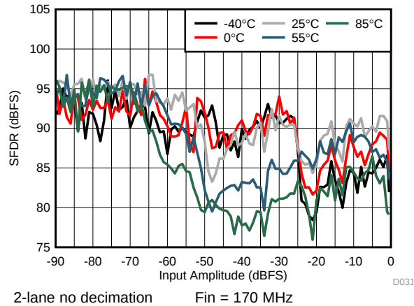
图 35. SFDR vs Amplitude
