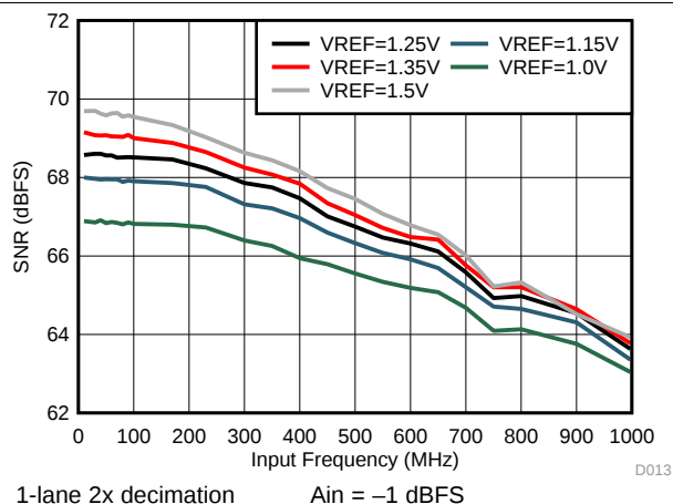
17. SNR vs. VREF
