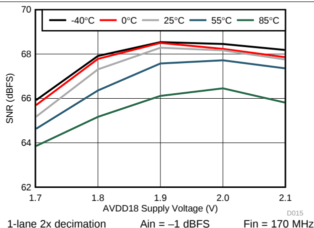
19. SNR vs. AVDD18
