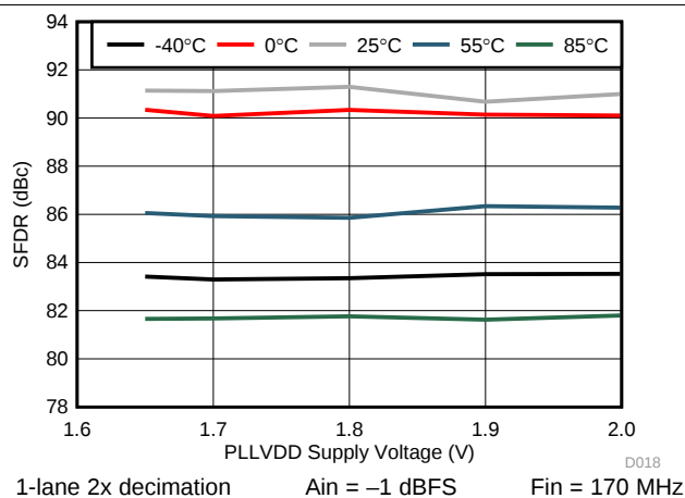
22. SFDR vs. PLLVDD
