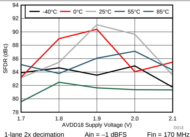
18. SFDR vs. AVDD18
