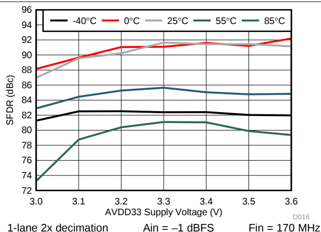
20. SFDR vs. AVDD33
