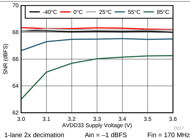
21. SNR vs. AVDD33
