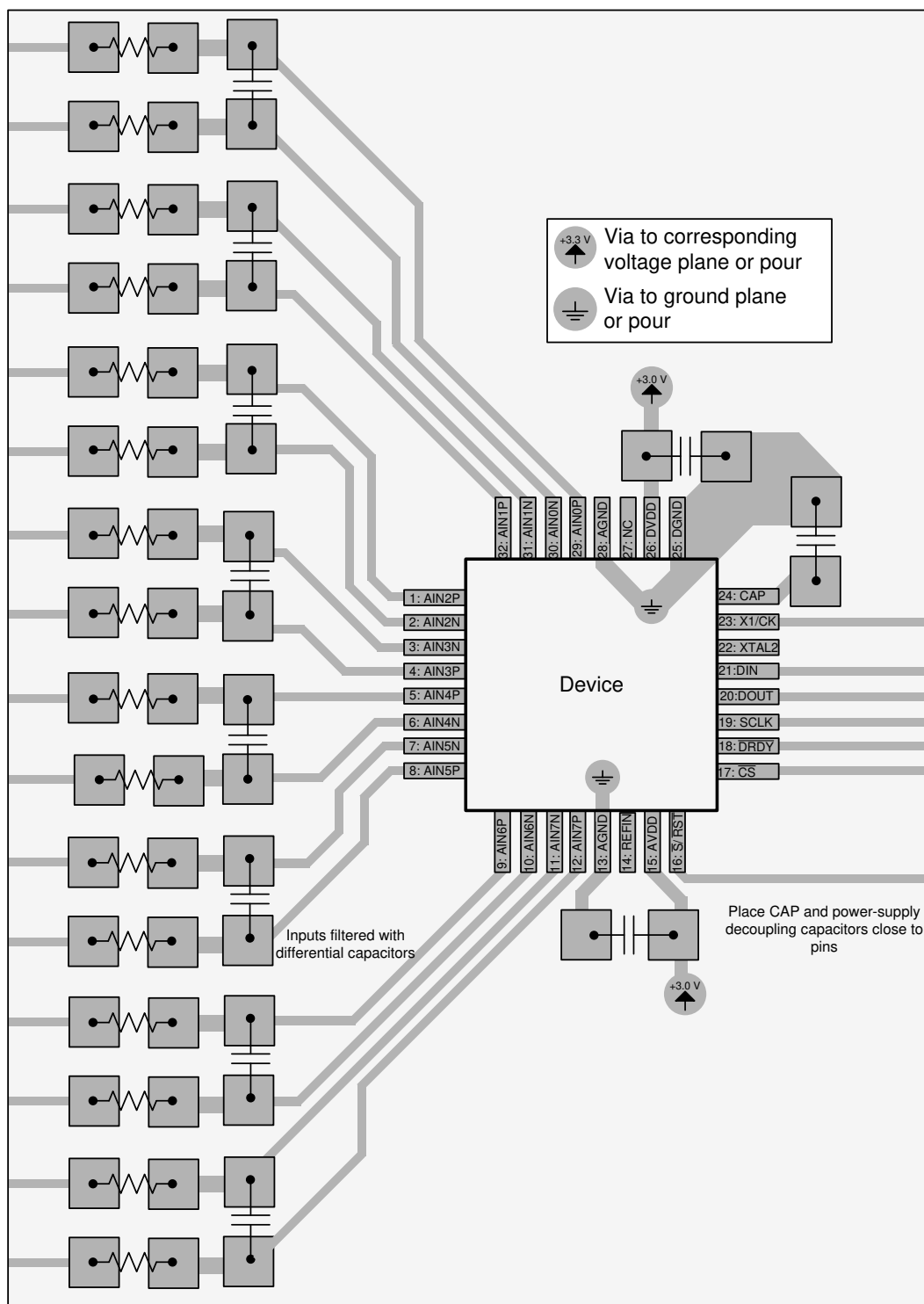
图 9-6. Layout Example
