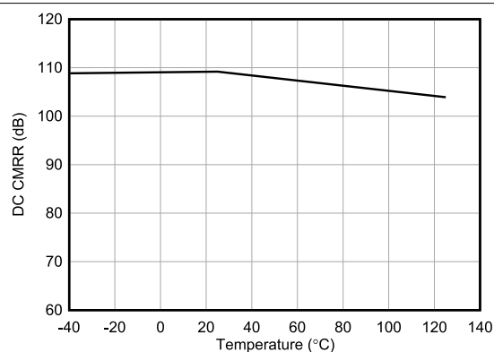
图 6-11. DC CMRR vs Temperature
