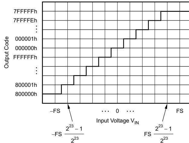
図 7-6. コード トランジション図 (24 ビットの変換データ)
