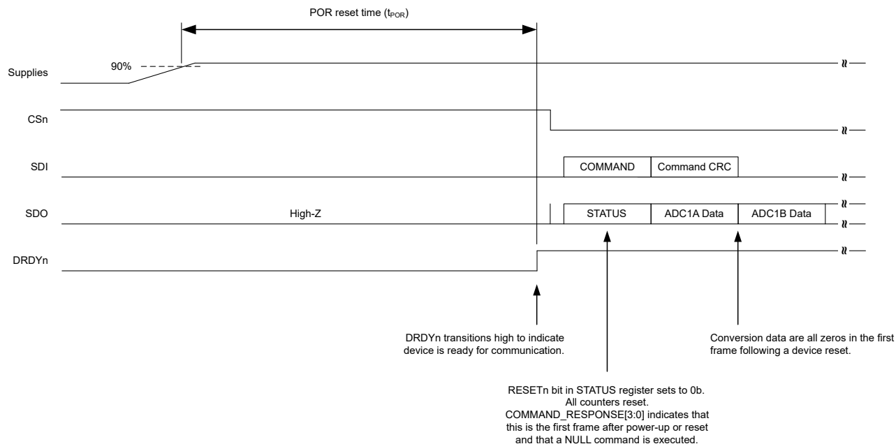
図 7-26. POR 後の DRDYn ピンの動作
