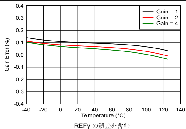
図 5-11. ADC2y のゲイン誤差と温度との関係
