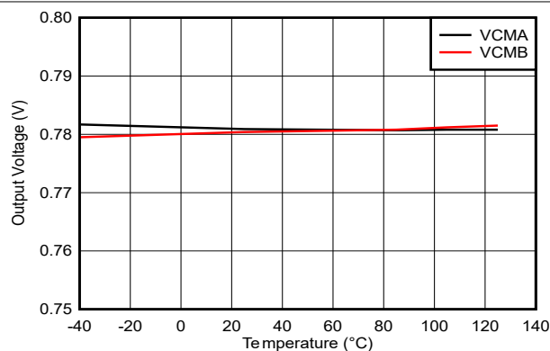
図 5-32. VCMx 出力電圧と温度との関係
