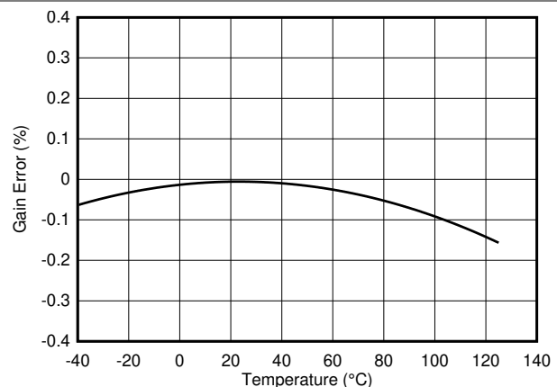
图 9-6. Gain Error vs Temperature
