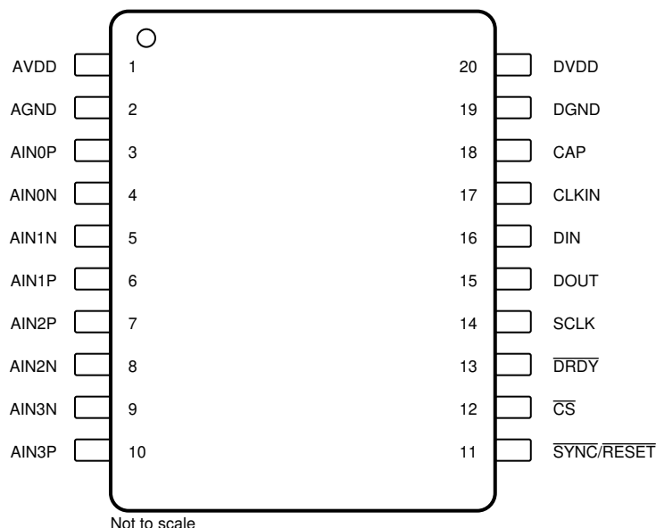
图 5-1. PW Package, 20-Pin TSSOP (Top View)
