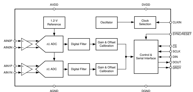
ブロック概略図
