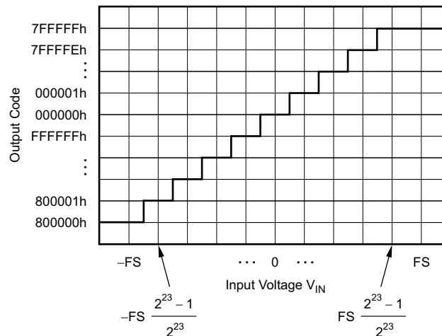
図 56. Code Transition Diagram
