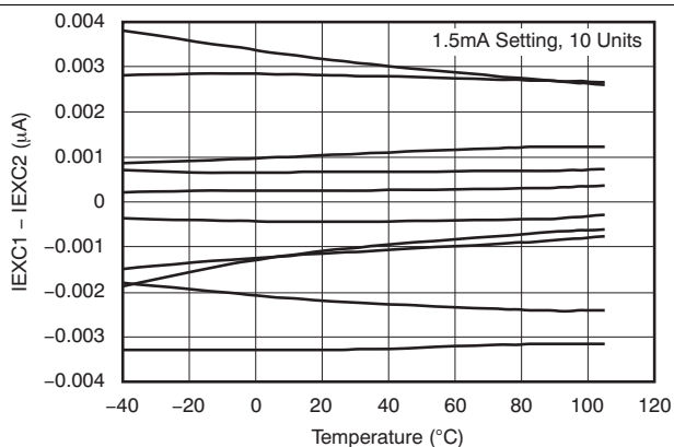
FIG 8. IDAC Drift
