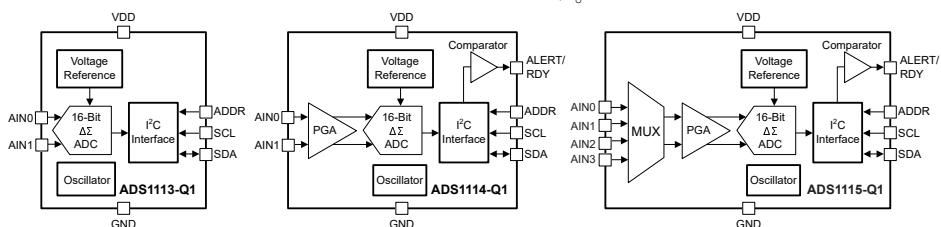
概略ブロック図
